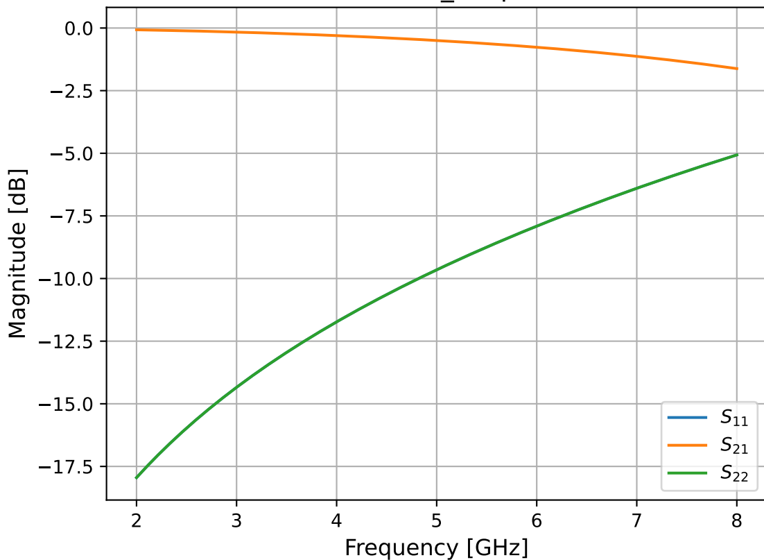
transmon_coupled
